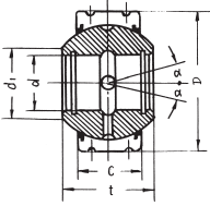
GEK...XS-2RS
