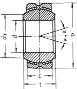
GEBK...S
